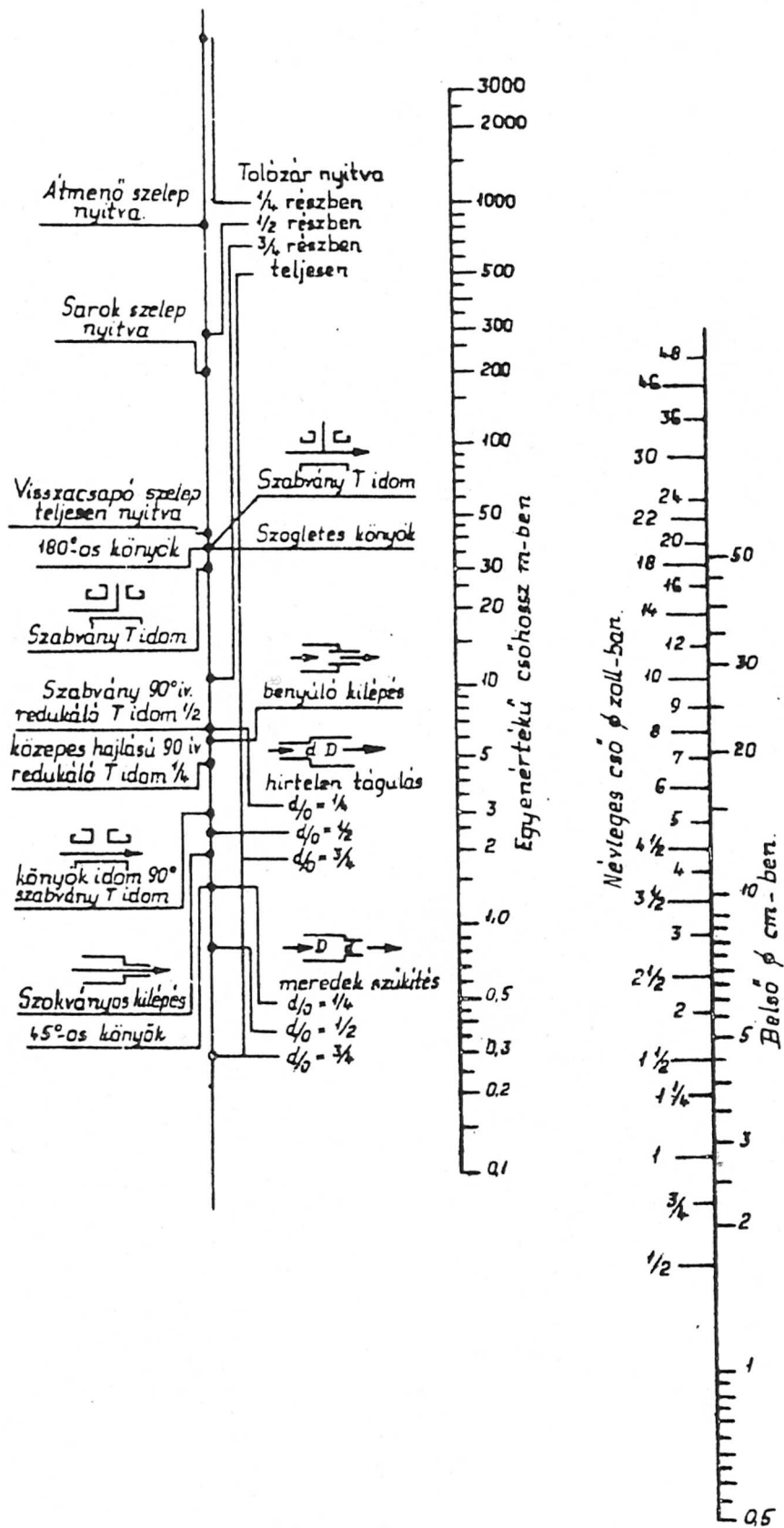
9.1. ábra Idomok, szerelvények egyenértékű csőhossza
