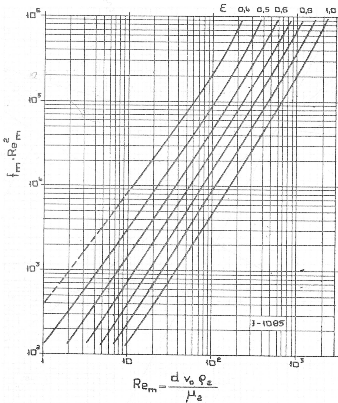
9.6. ábra Töltött oszlopok f_m Re_m^2 - Re_m diagram
