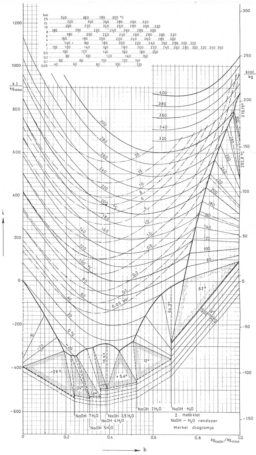
9.12. ábra NaOH – H 2 O rendszer Merkel diagramja
